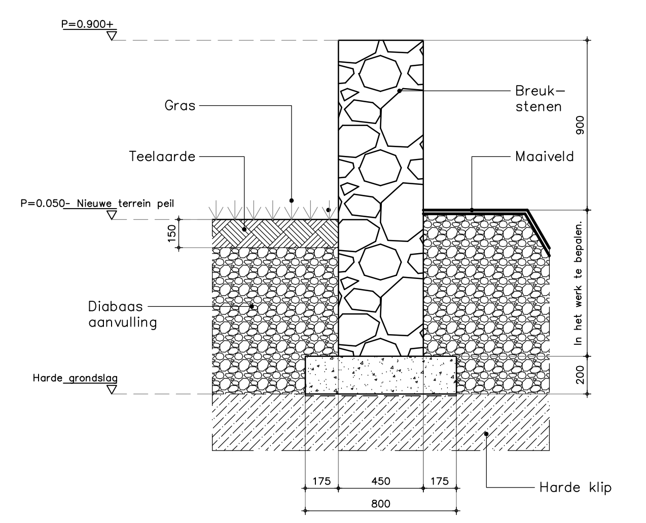
PRINCIPE DETAIL 02
