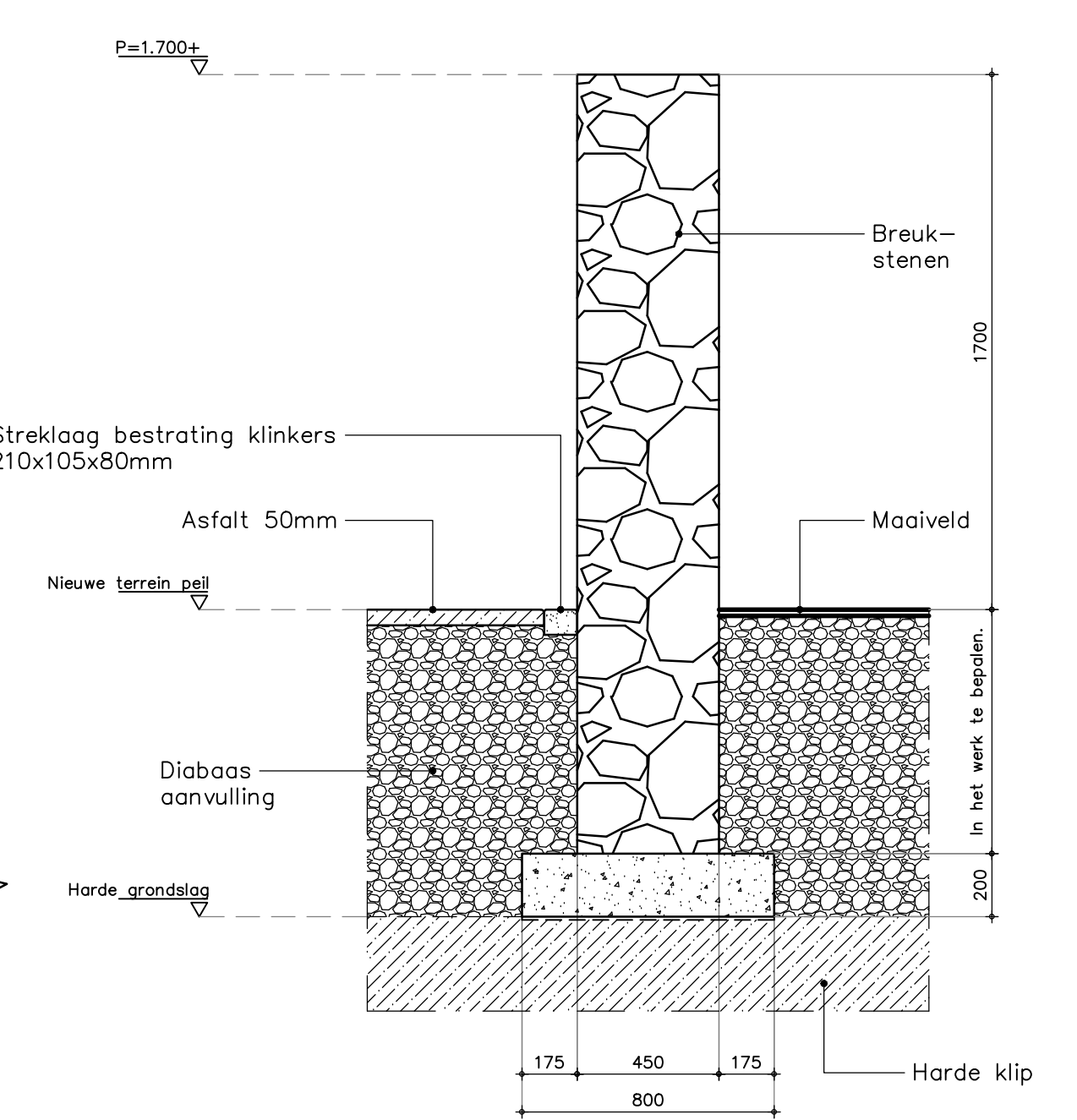
PRINCIPE DETAIL 01
